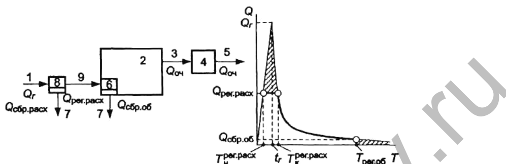
Рис. 2. Принципиальная схема разделения дождевого стока перед очистными сооружениями и схематический расчетный гидрограф дождевого стока
