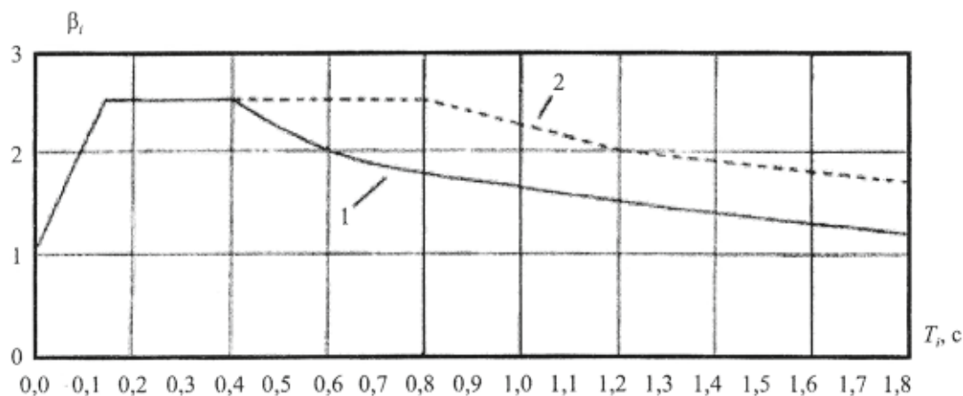
Рисунок 3 – Коэффициенты динамичности \beta(T_i)
